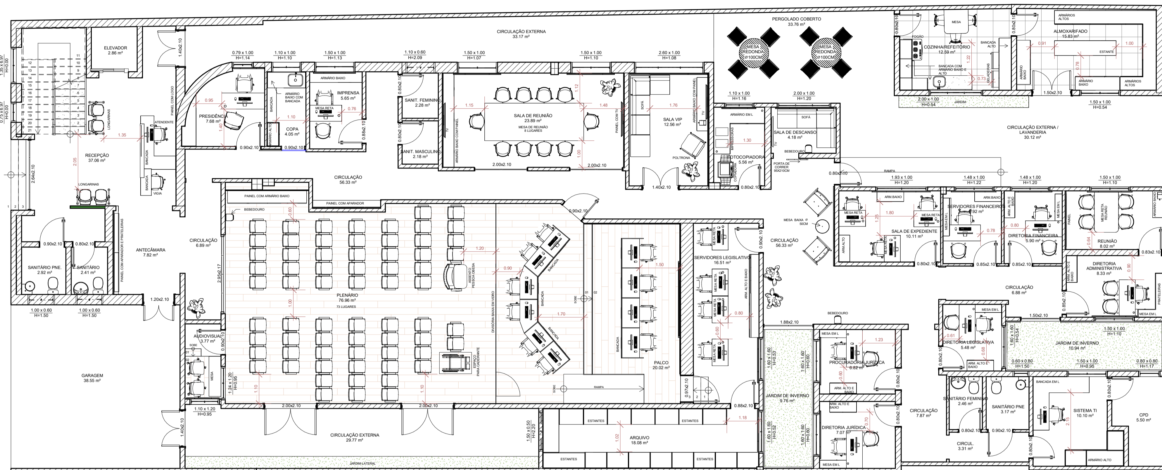
1 PLANTA DE LAYOUT - TÉRREO 1:75
